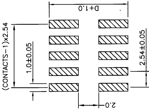
P.C.B SMD LAYOUT
