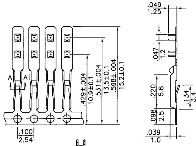
A-A SECTION
