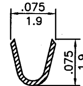
A-A SECTION
