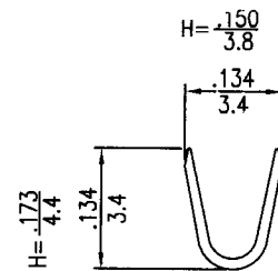
A-A SECTION
