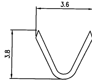
A-A SECTION
