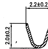
A-A SECTION
