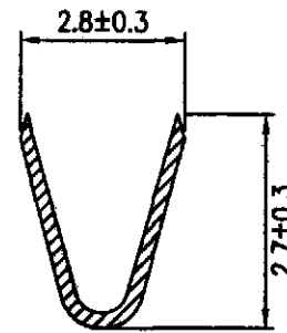
A-A SECTION
