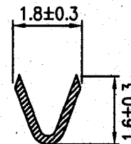
A-A SECTION
